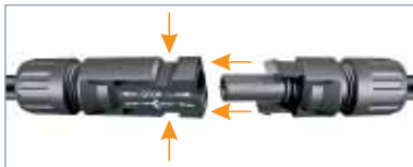
Verriegelungssystem Locking system Système de verrouillage
