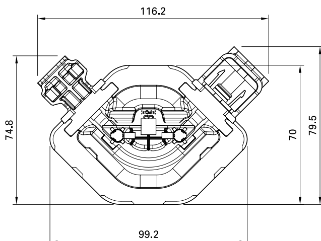
Moduleseitige Lötanschlüsse Solder connections on module Bornes à souder sur le module
