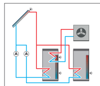
Système de chauffage solaire à 2 réservoirs, logique de pompe et chauffage d'appoint à travers une pompe à chaleur
