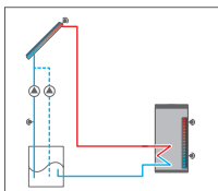
Système drainback avec pompe booster*
