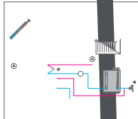
Système de chauffage solaire à 1 réservoir, augmentation de la température de retour dans le circuit de chauffage et chauffage d'appoint thermostaté
