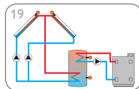
Système de chauffage solaire avec capteurs est/ouest et chauffage d'appoint (p. 28)
