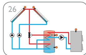
Système de chauffage solaire avec capteurs est/ouest et chaudière à combustible solide (p. 35)
