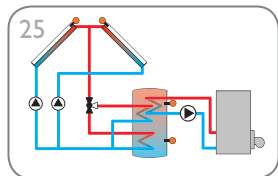
Système de chauffage solaire avec capteurs est/ouest et chauffage d'appoint (p. 34)
