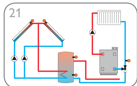
Système de chauffage solaire avec capteurs est/ouest et augmentation de la température de retour (p. 30)
