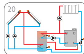
Système de chauffage solaire avec capteurs est/ouest, augmentation de la température de retour et chauffage d'appoint (p. 29)
