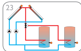
Système de chauffage solaire avec capteurs est/ouest, 2 réservoirs et logique de vanne (p. 32)
