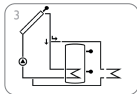
Système de chauffage solaire standard avec évacuation de l'excès de chaleur (page 17)
