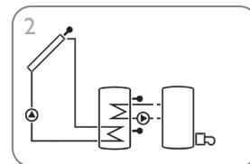
Système de chauffage solaire avec chauffage d'appoint (page 12)
