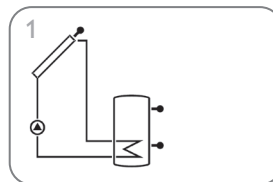
Système de chauffage solaire standard (page 9)
