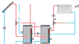
Système à 2 réservoirs, commande pompe circulation, chaudière combustible solide et circuit de chauffage dépendant des conditions climatiques
