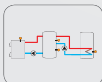
Chaudière à combustible solide avec fonction échange de chaleur
