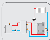
Chaudière à combustible solide avec augmentation de la température du retour
