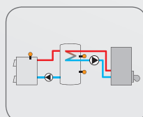
Chaudière à combustible solide avec chauffage d'appoint thermostatique
