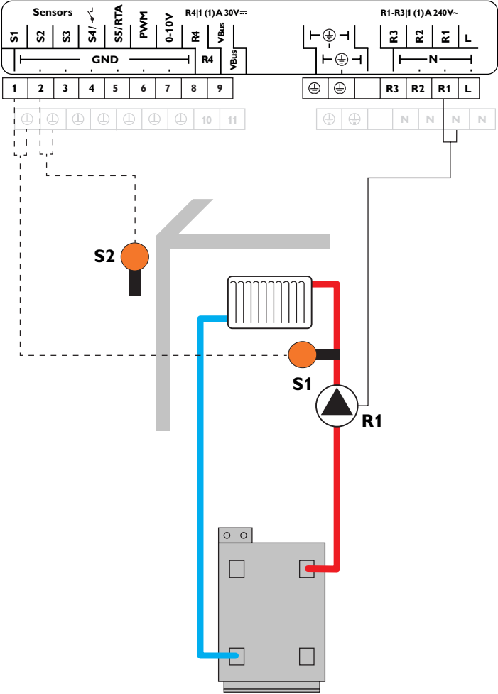
Schéma 3: circuit de chauffage direct
