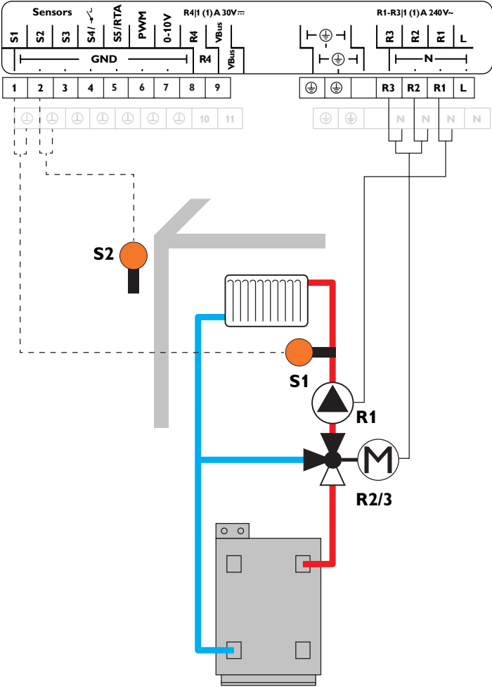
Schéma 1: circuit de chauffage mélangé
