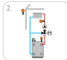
1 circuit de chauffage mélangé avec chauffage d'appoint (demande) (voir page 20)
