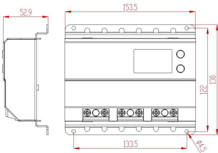
Pic.5 Dimensions
